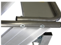
Las barandillas se atornillan en la parte superior de los perfiles
