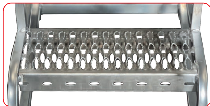
Gradini in alluminio grigliato (optional): supergrip e drenanti per olio, cemento e neve
