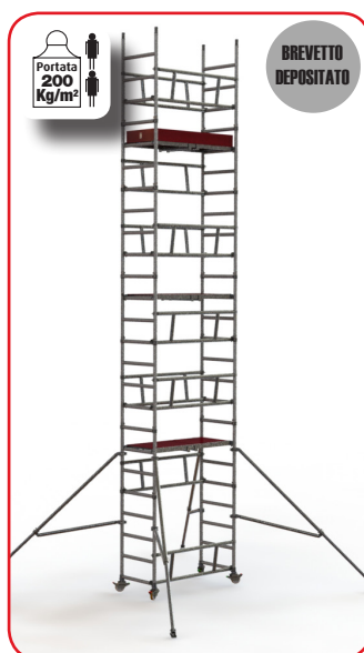
SVELTOWER montato alla massima altezza m 5,67
