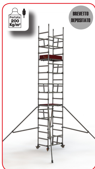
SVELTOWER montato alla massima altezza m 5,67
